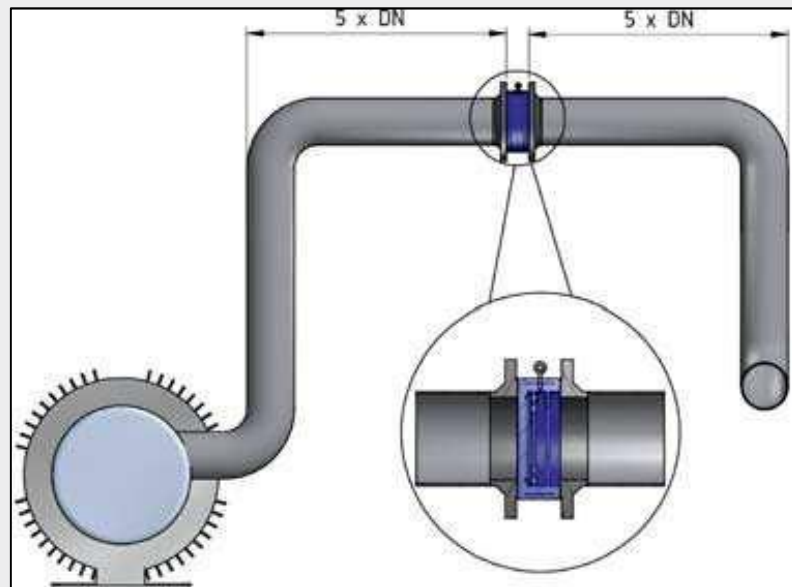
(ABB. 1 / pic. 1) Leitungsbeispiel / Pipeline example
